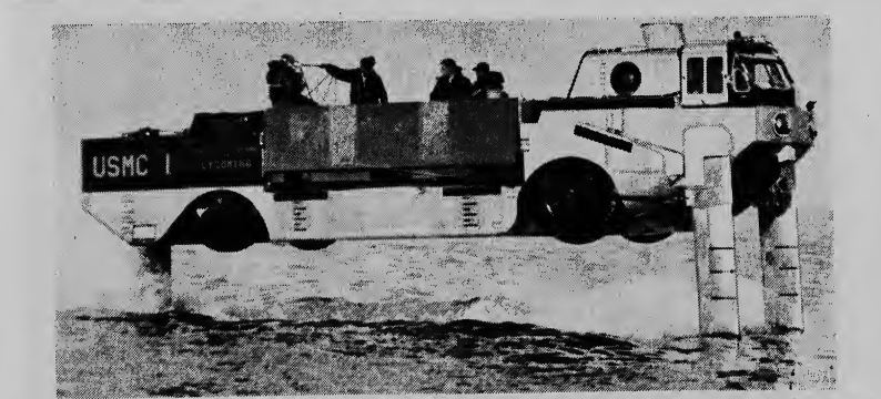
E aparato aki na un LVH, qu a ser construi pa AVCO, riba orden di U.S. Marine Corps. Actualmenten nan ta ponela a prueba na Pendleton, California.
